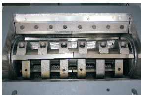
RG-26E/36E 片刀型 Paddle blades type
