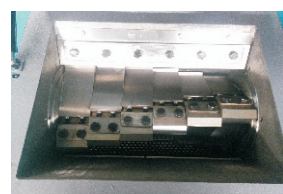
RG-26EB/36EB 平刀型 Flat blades type
