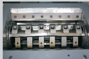
RG-66S Paddle blades type
